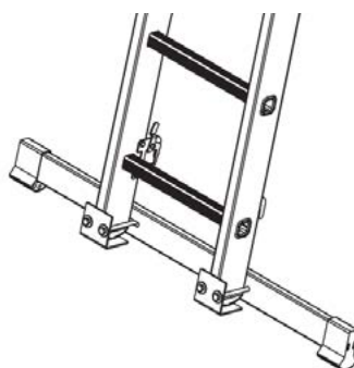
Stabilisateur 900 [mm]
